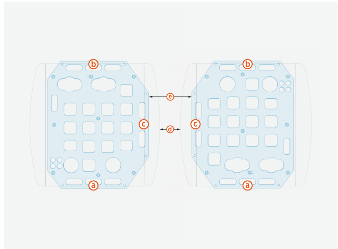
Deux Power Blocks disposés dos à dos
